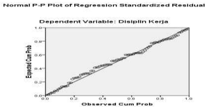
Gambar IV.1 Uji Normalitas
