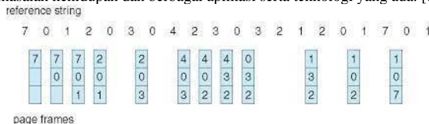
Gambar 1. Algoritma FIFO
